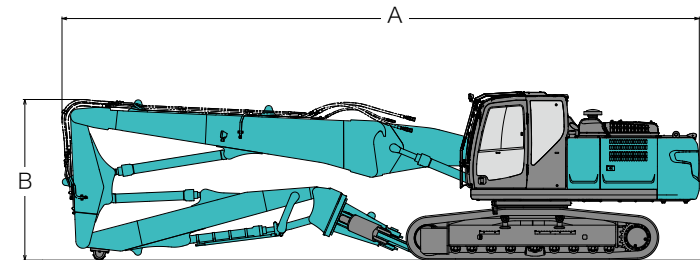
3 っ折れ超ロングアタッチメント仕様
