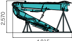
■2っ折れ超ロングアタッチメント
