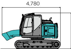
■本体+メインブーム
