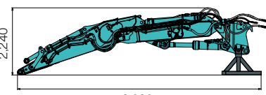
■セバレートブームアタッチメント
