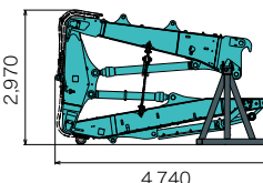
■3っ折れ超ロングアタッチメント
