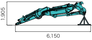
■セバレートブームアタッチメント
