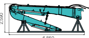
■2っ折れ超ロングアタッチメント
