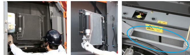
防塵ネット 開閉式エアコンデンサ ラジエータ清掃窓
